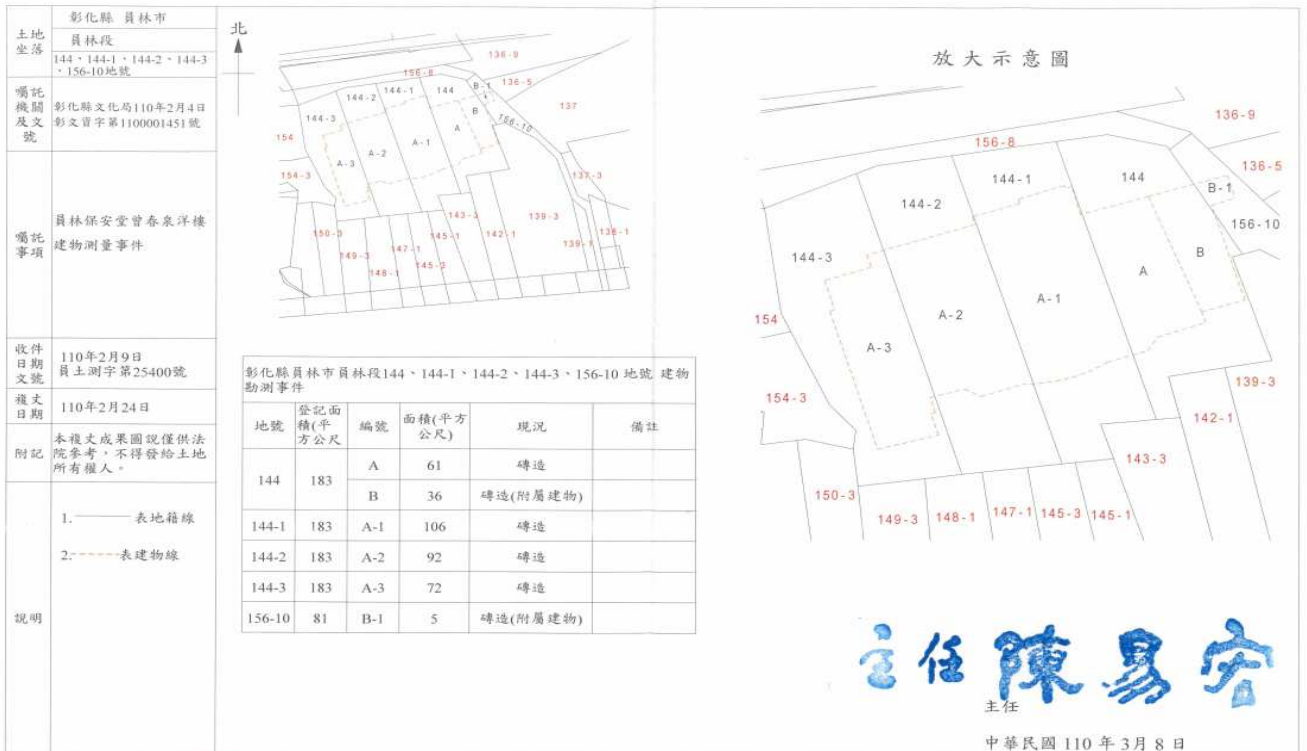
彰化縣員林地政事務所土地複丈成果圖
